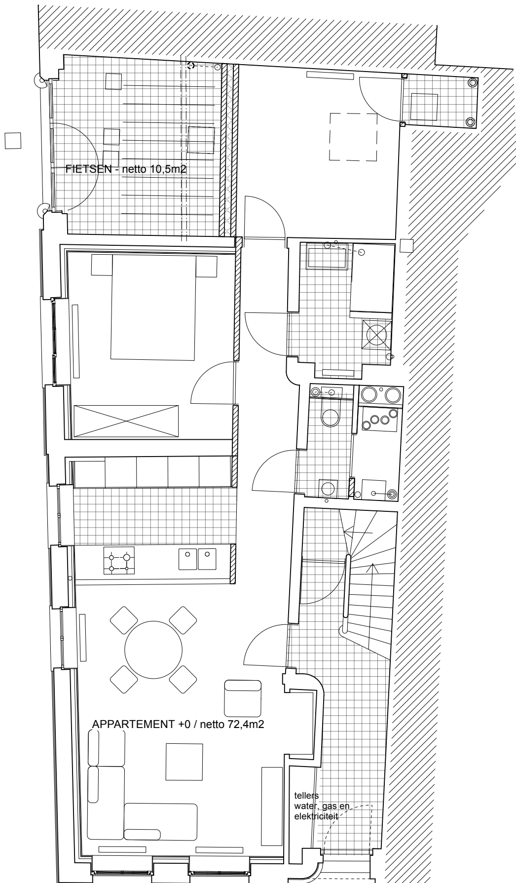
APPARTEMENT GELIJKVLOERS (n° 32)
